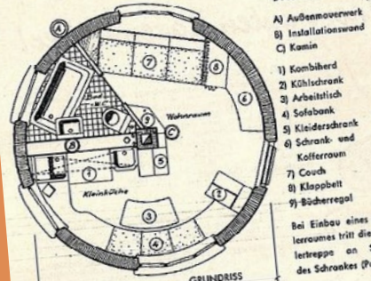
> Plattegrond van Ludowici's bolwoning uit de jaren 60.
